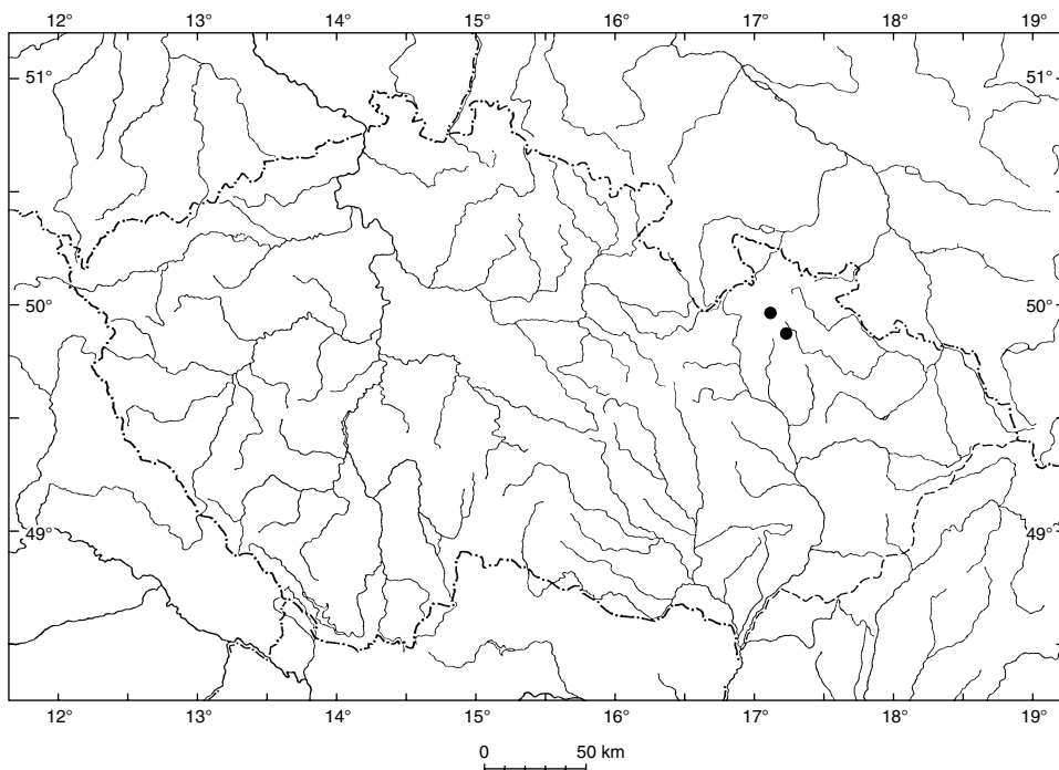
Fig. 2. Distribution of Cynodontium gracilescens (F.WEBER et D. MOHR) SCHIMP.
