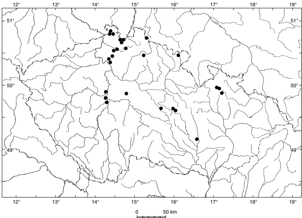
Fig. 3. Distribution of Cynodontium tenellum (BRUCH, SCHIMP. et GÜMBEL) LIMPR.
