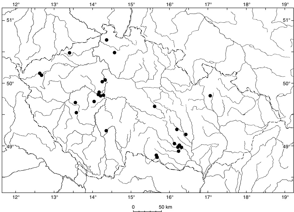
Fig. 1. Distribution of Cynodontium bruntonii (SM.) BRUCH et SCHIMP.
